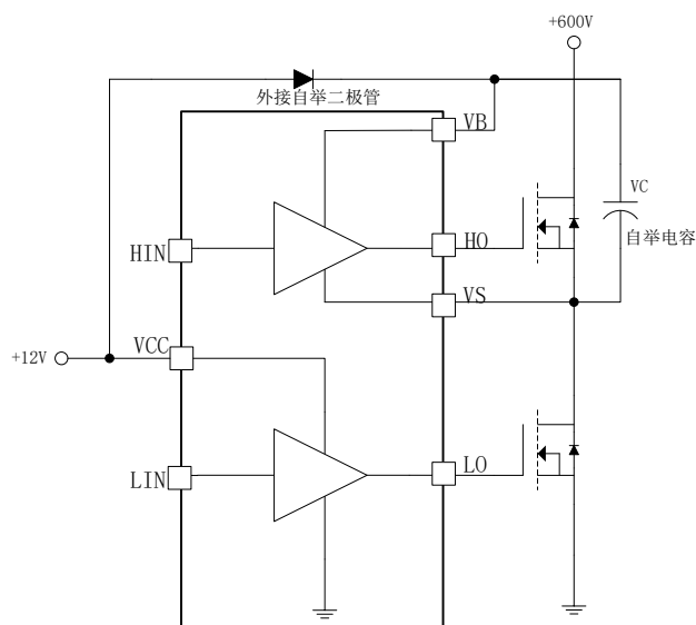
图 8-3. EG2304 自举电路结构
