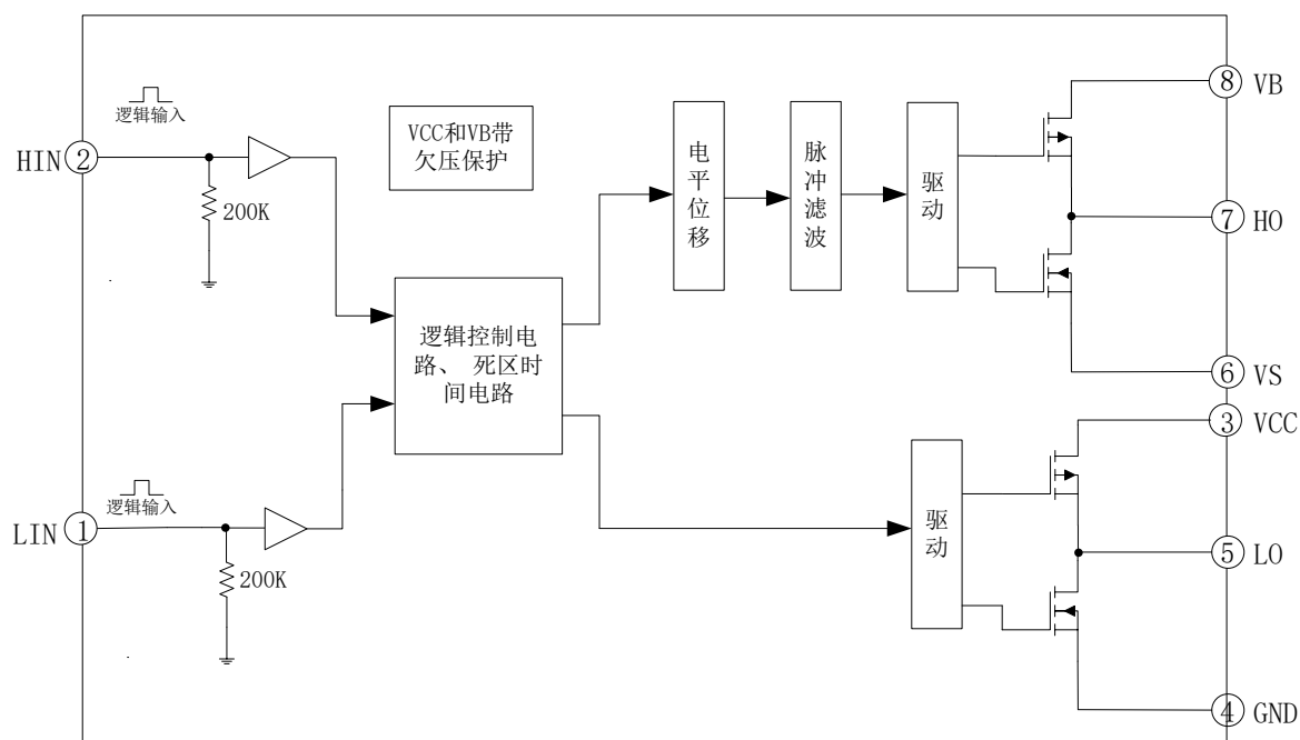
图 5-1. EG2304 内部电路图
