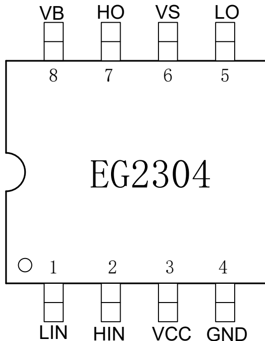
图 4-1. EG2304 管脚定义
